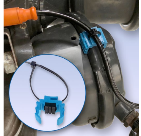
Sujetacables WABCO
