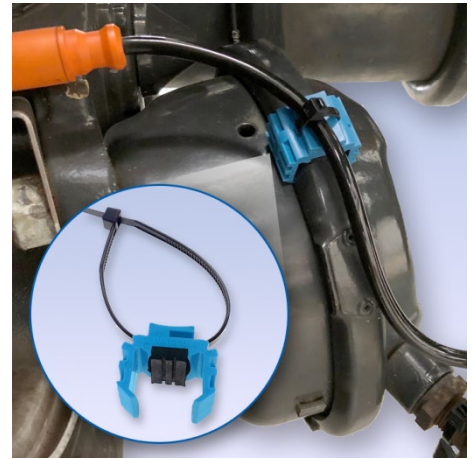
WABCO kabelbevestigingsklem
