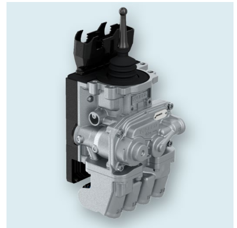
WABCO Central Braking Unit (CBU) 480 020 028 0
