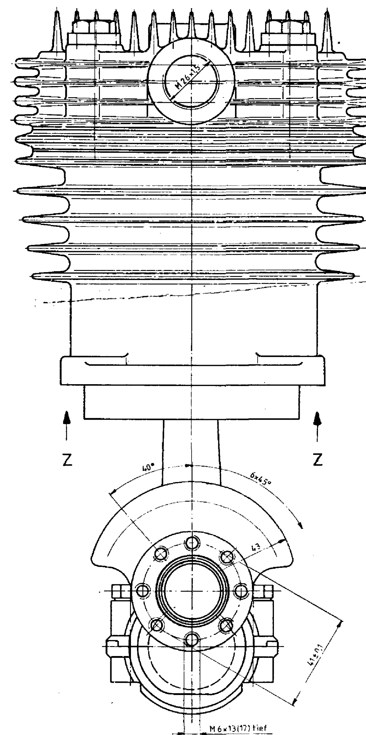
Ansicht Z
