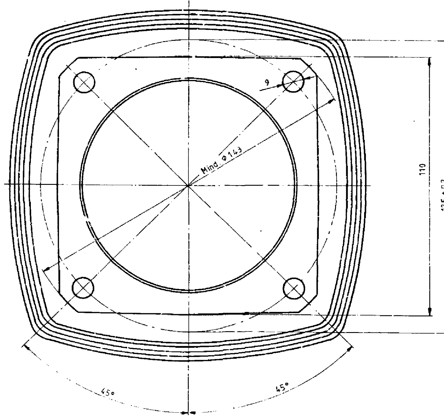
Ansicht Z
