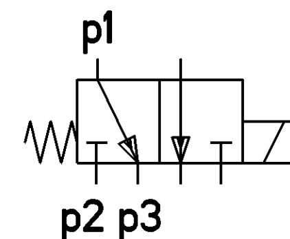
FUNCTION SCHEME/ FUNKTIONSSCHEMA
