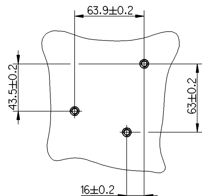
CONNECTING HOLE PATTERN ANSCHLUSSLOCHBILD
