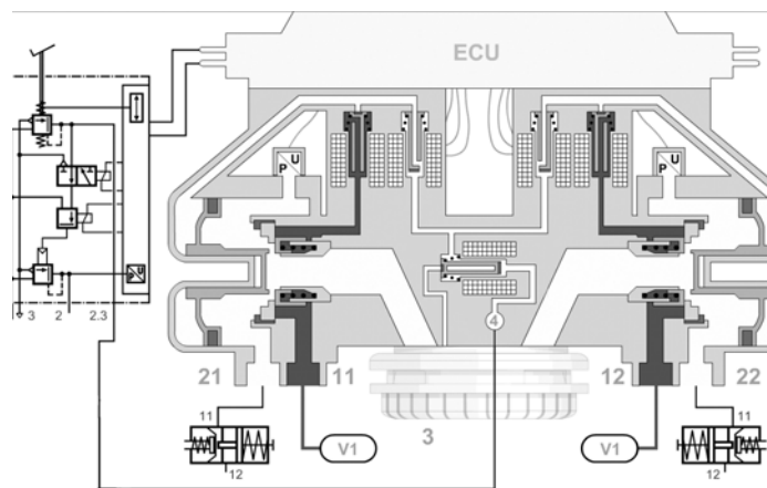
Рис. 28: Принцип действия модулятора оси 3-ого поколения
