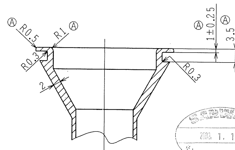
A部詳細 (2:1)
