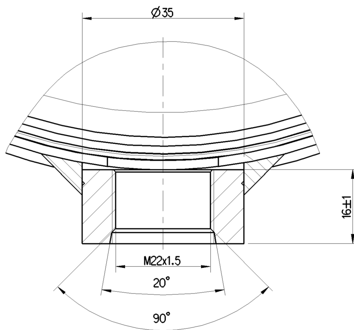
A 2:1 4-PLACES
