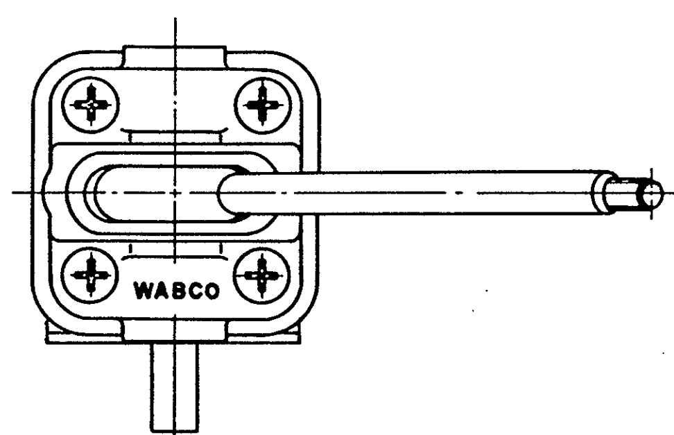
VISTA SUPERIOR SEM SANFONA E PUNHO VIEW W/O BOOT AND HANDLE
