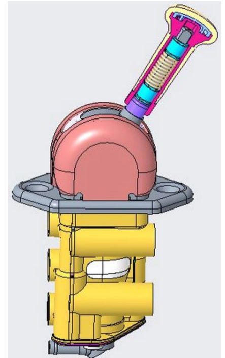
Slika 1: Ventil ručne kočnice
