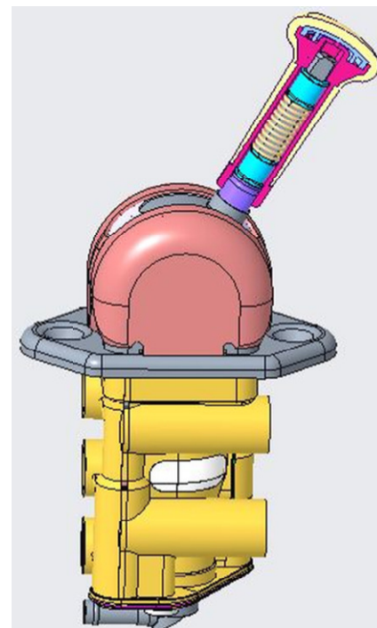
Obrázek 1: Ventil ruční brzdy
