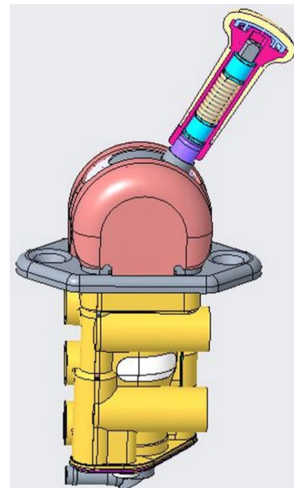
Slika 1: Ventil ručne kočnice
