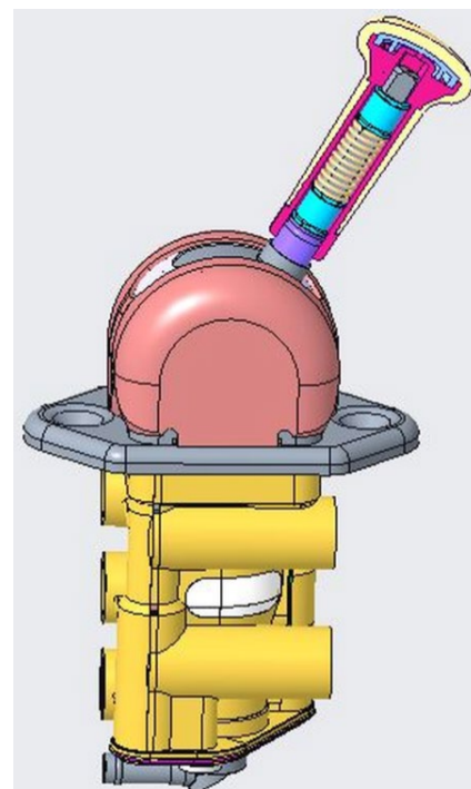
1. kép: Kézifékszelep
