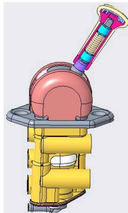
図1: ハンドブレーキ・バルブ
