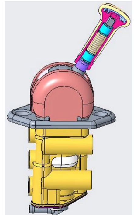
Bild 1: Handbromsventil
