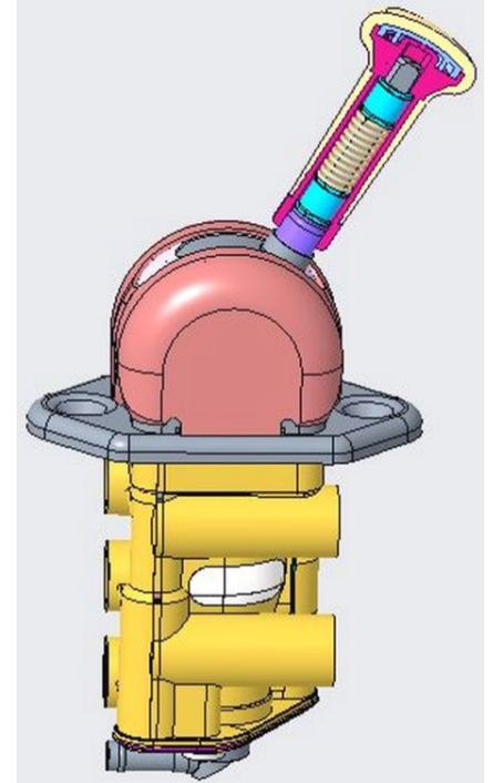
Resim 1: El freni valfi
