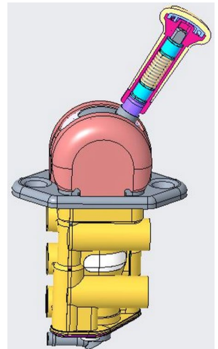
Малюнок 1: клапан ручного гальма
